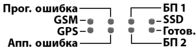
Рисунок 7 – Светодиодная индикация и порты передней панели УСПД
