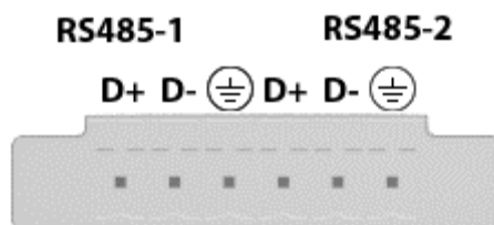
Рисунок 5 – Маркировка клемм RS-485
