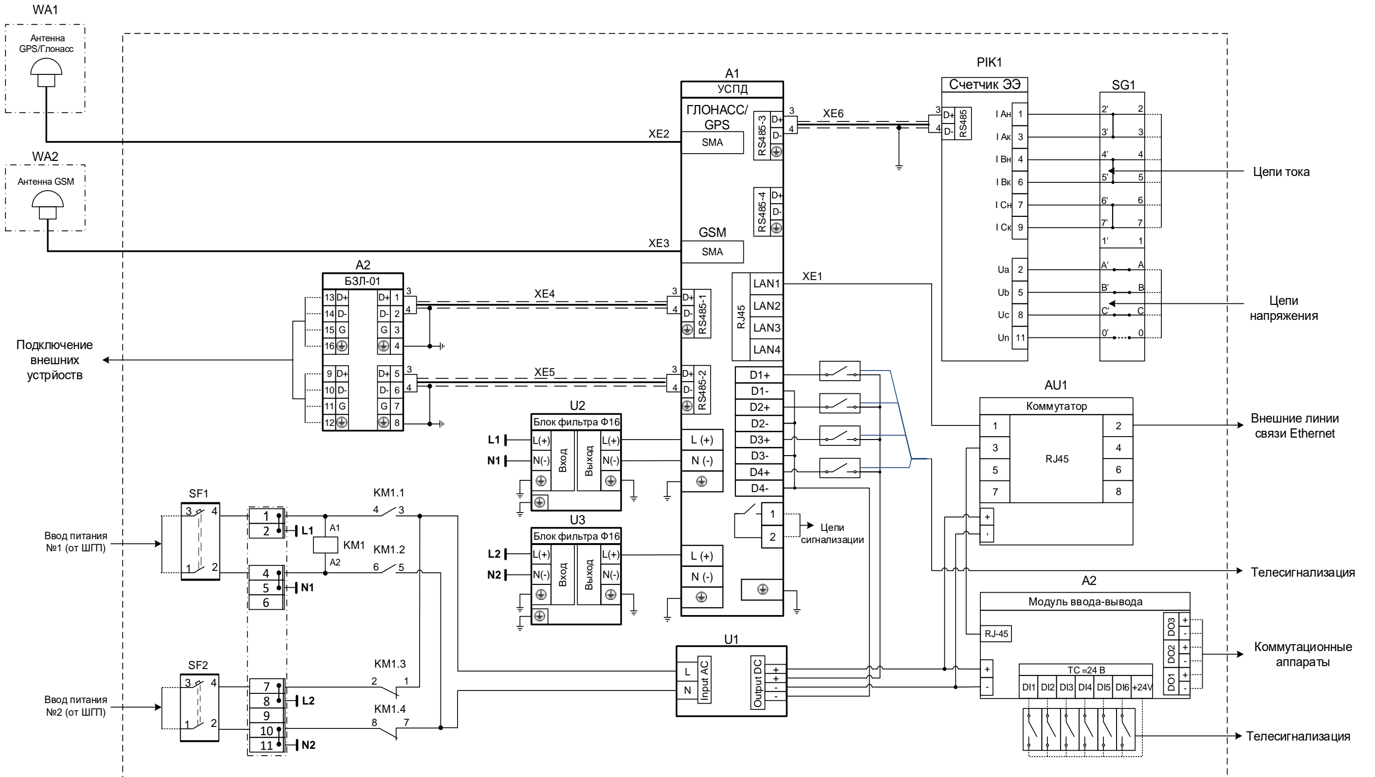
Рисунок Д.2 – Пример подключения внешних устройств к УСПД в составе шкафа
